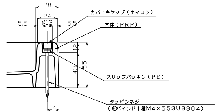
A-A断面図1/2
