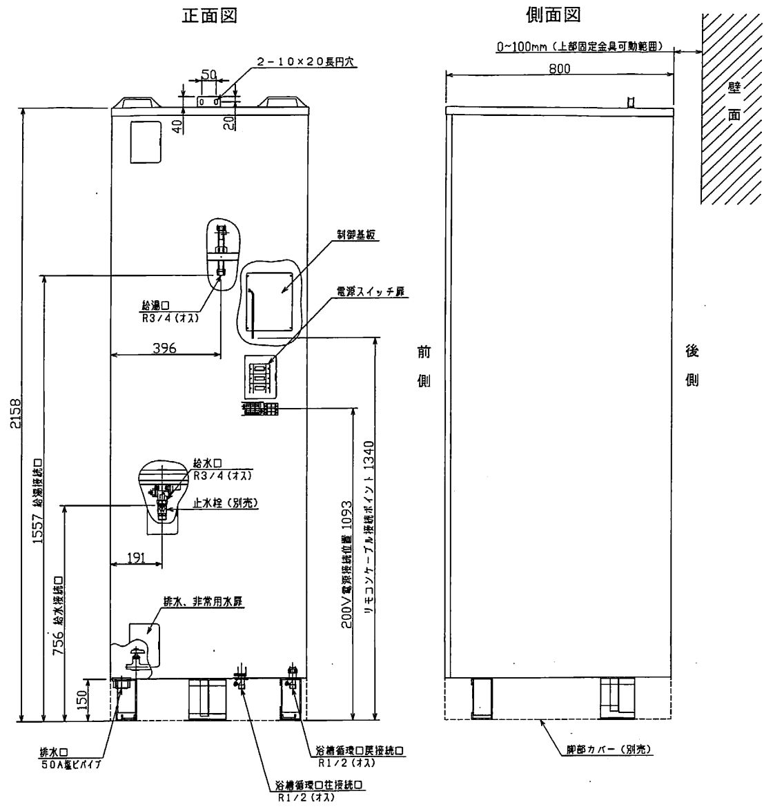
配管、配線用穴、アンカーボルト位置図
