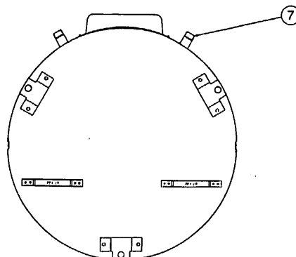
B部詳細
