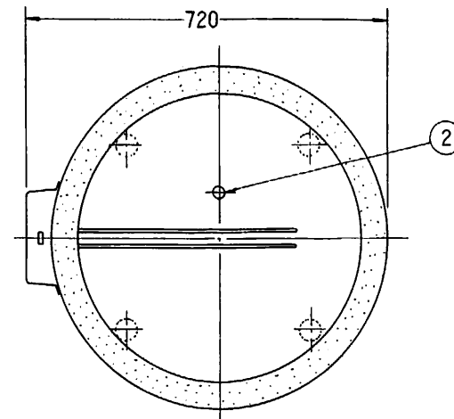
A-A' 断面図
