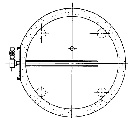
A-A 断面図
