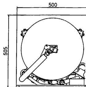
A-A断面図
