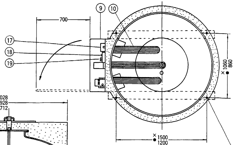
A-A' 断面図 アンカーボルト取付穴20φ
