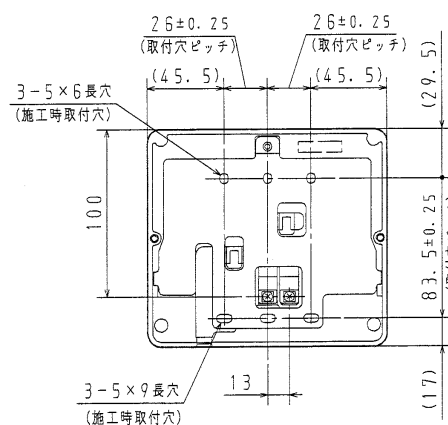
リモコン取付台寸法図 (裏面)
