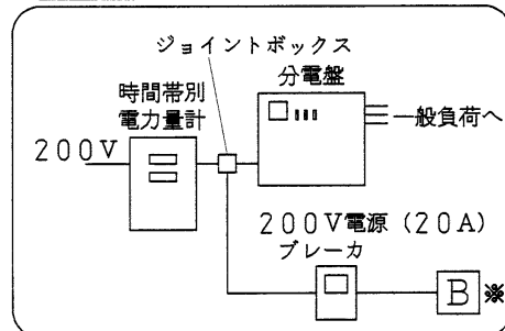
貯湯タンクユニット「200V電源線、ヒートポンプ電源線、リモコン線」配線図
