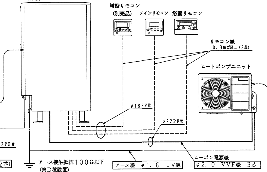
ヒートポンプユニット 「ヒートポンプ電源線、アース」配線図
