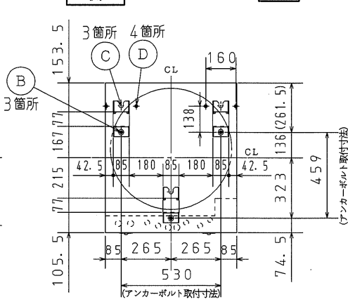
アンカーボルト位置図
