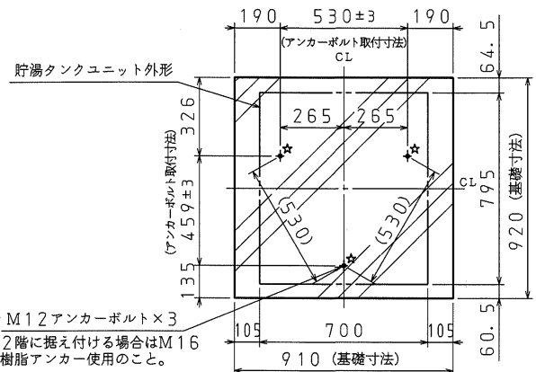
独立基礎の場合のアンカーボルト位置図 (参考)
