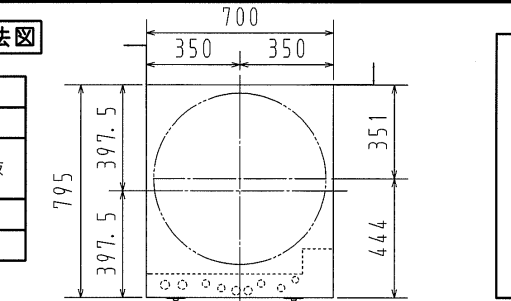
上面
