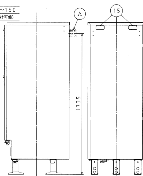
右側面
