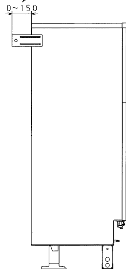
左側面
