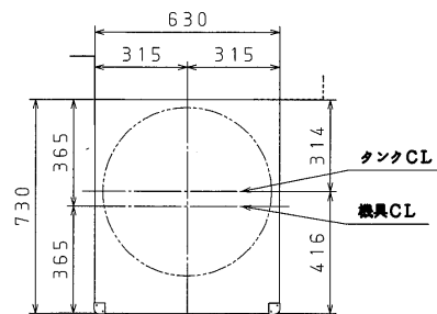
上面
