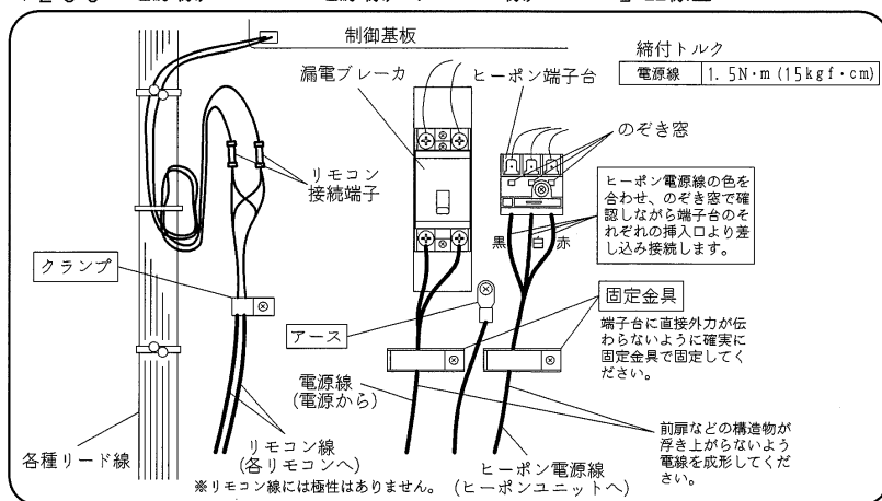
制御ユニット 「200V電源線、ヒーポン電源線、リモコン線、アース」配線図
