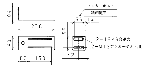
壁固定金具 外形寸法図
