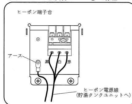
ヒートポンプユニット 「ヒーポン電源線、アース」配線図
