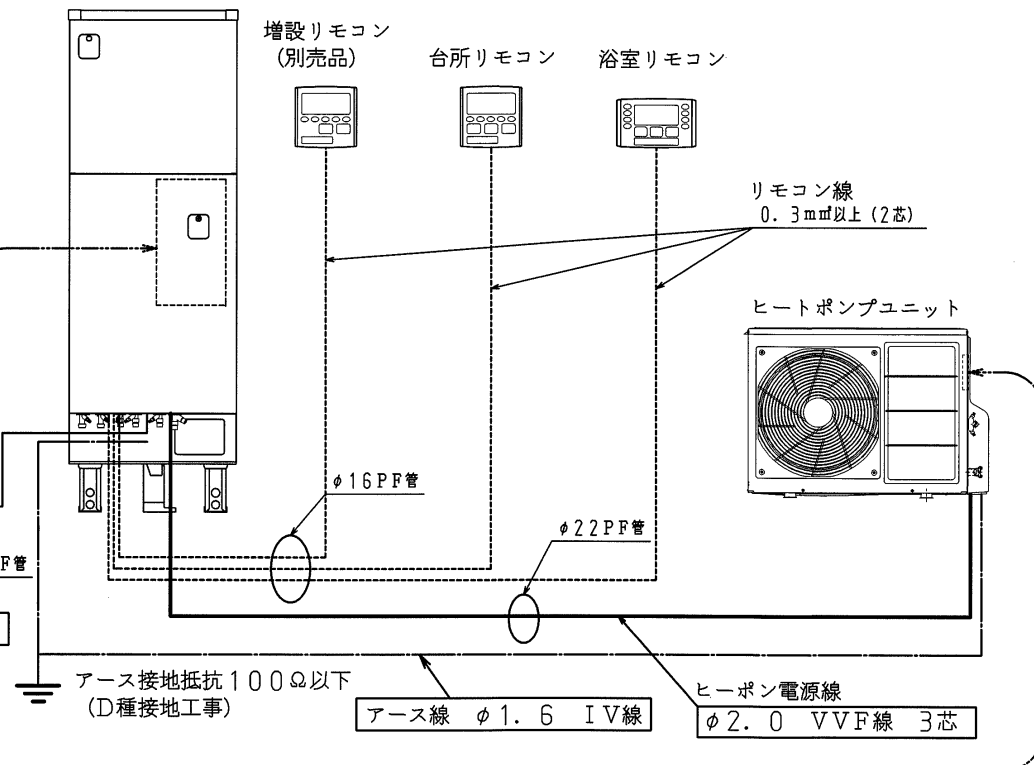
貯湯タンクユニット
