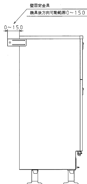
左側面
