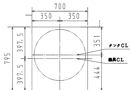
上面
