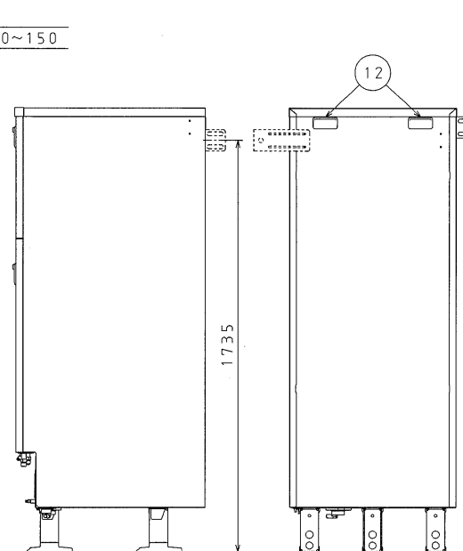
右側面
