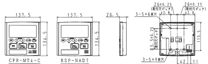
リモコン取付寸法図 (裏面)
