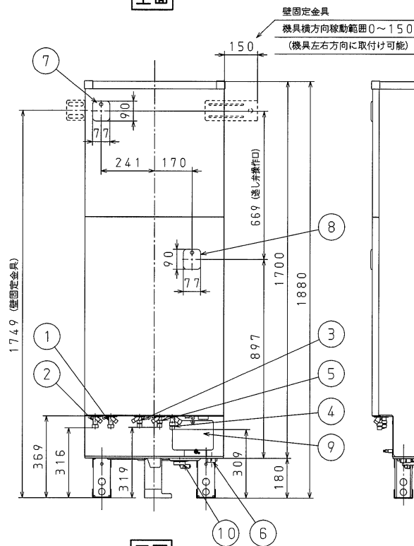
正面
