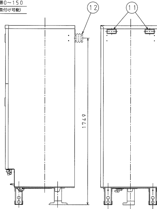
右側面
