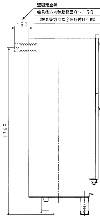
左側面
