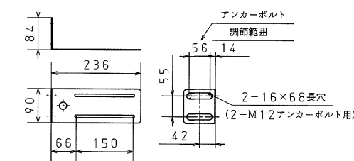
壁固定金具 外形寸法図 (本体に1個付属)
