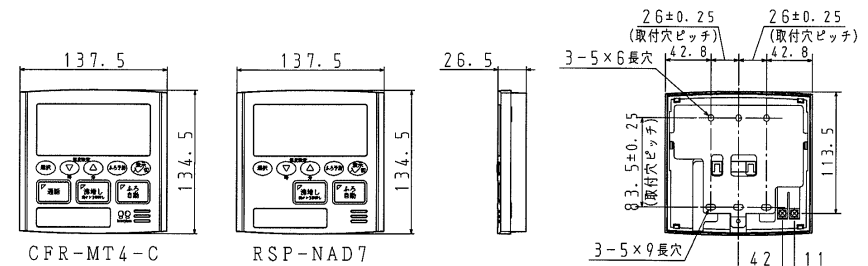
リモコン取付寸法図 (裏面)
