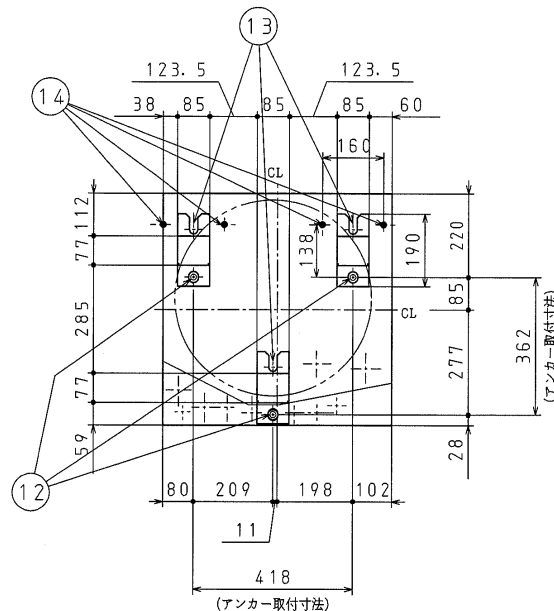
アンカー位置図
