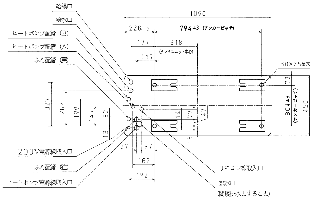
配線・配管立上げ位置図
