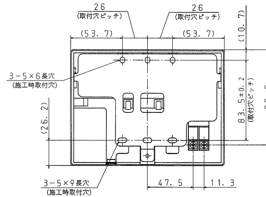
リモコン取付寸法図 (裏面)
