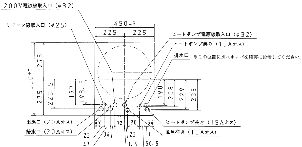
配管寸法図
