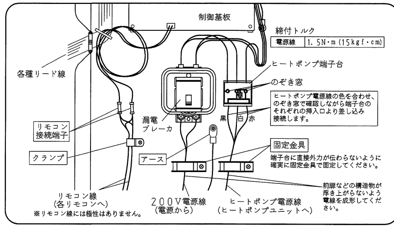
貯湯タンクユニット 「200V電源線、ヒートポンプ電源線、リモコン線、アース」配線図
