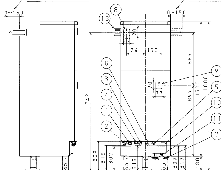
左側面
