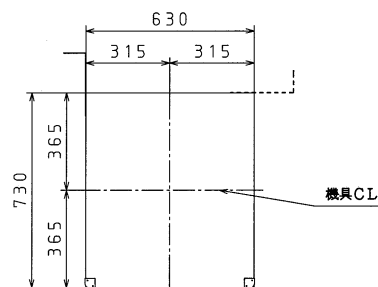
上面
