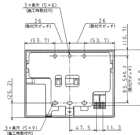
リモコン取付寸法図 (裏面)
