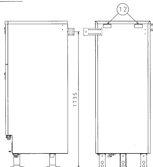
背面
