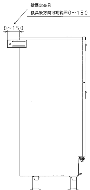
左側面
