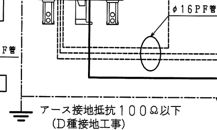
ヒートポンプユニット 「ヒートポンプ電源線、アース」配線図
