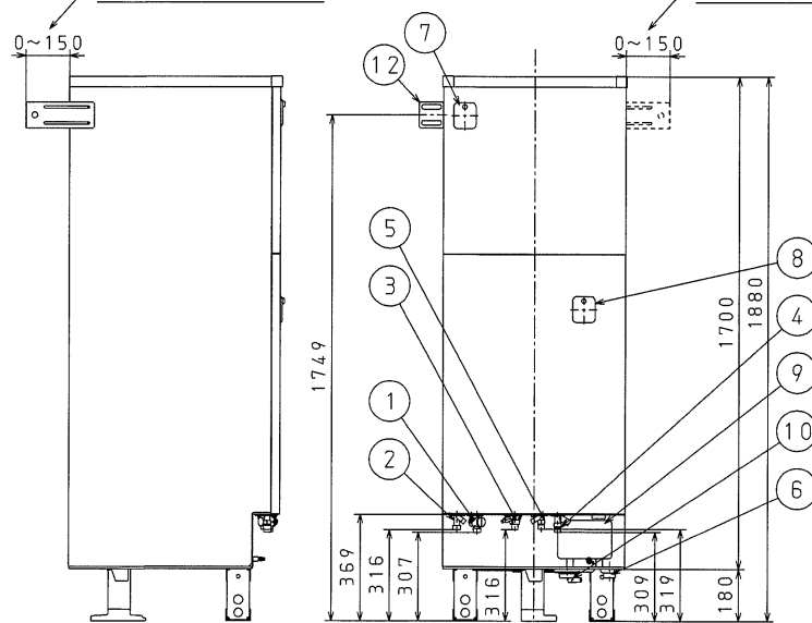
左側面
