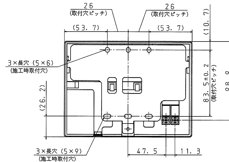
リモコン取付台寸法図 (裏面)
