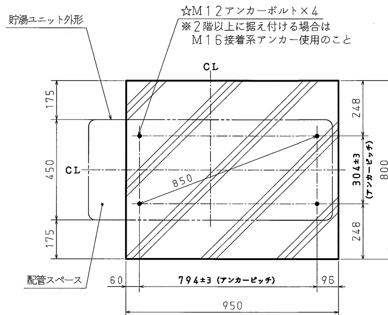
独立基礎の場合のアンカー位置図 (参考)
