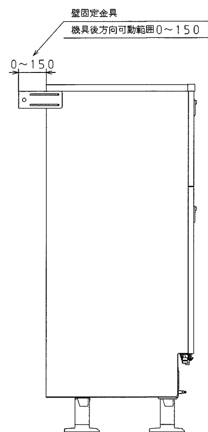
左側面
