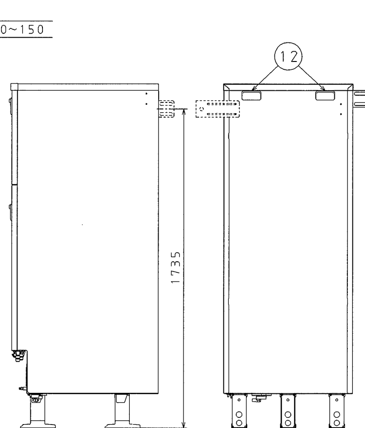
背面
