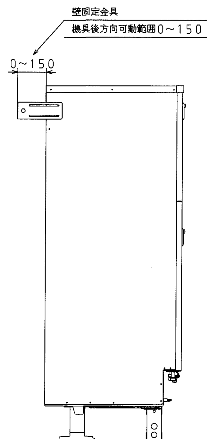
左側面
