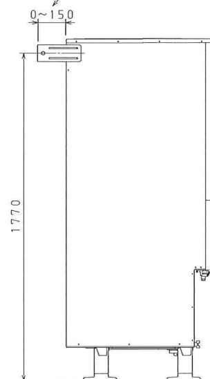
左側面
