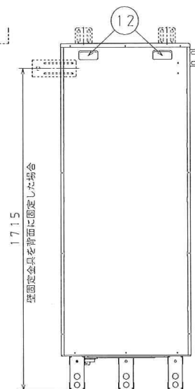
背面
