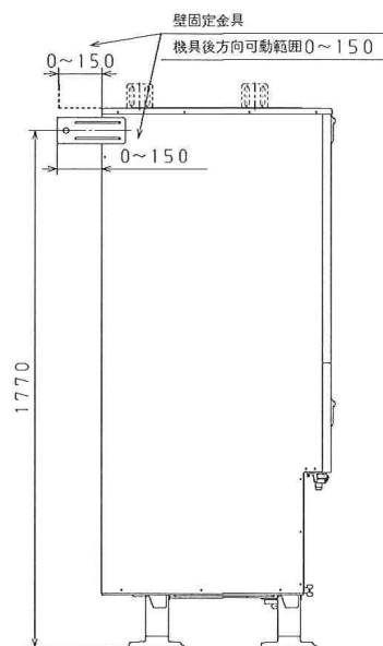
左側面
