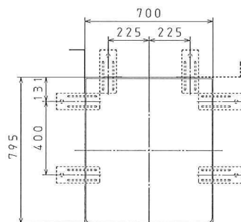
上面
