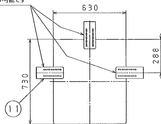
上面
